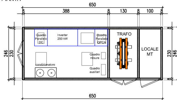
PIANTA
