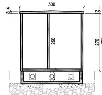
SEZIONE
