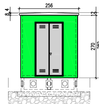
PROSPETTO P4
