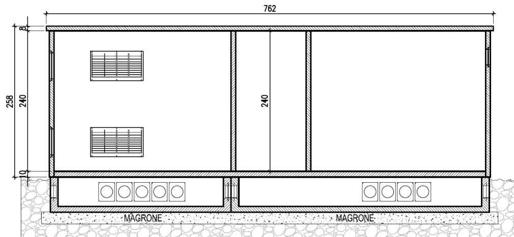
SEZIONE A-A
