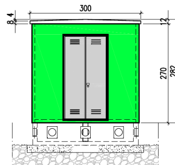
PROSPETTO P4
