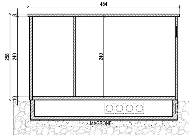
SEZIONE A-A
