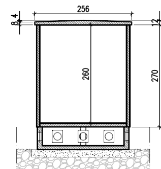
SEZIONE
