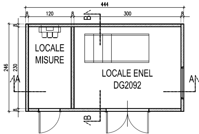
PIANTA SOLAIO
