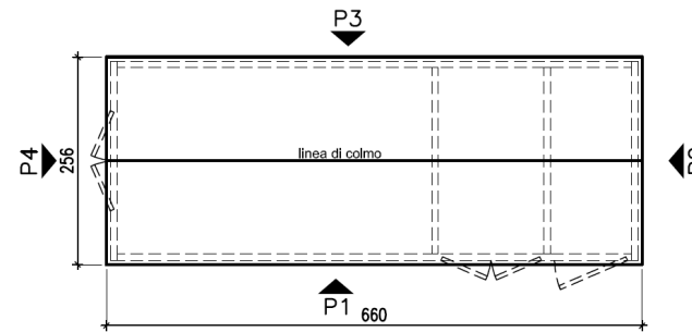
PIANTA COPERTURA
