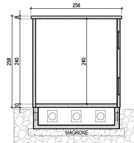
SEZIONE B-B
