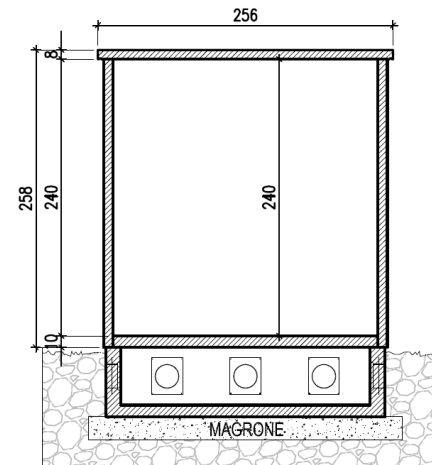
SEZIONE B-B
