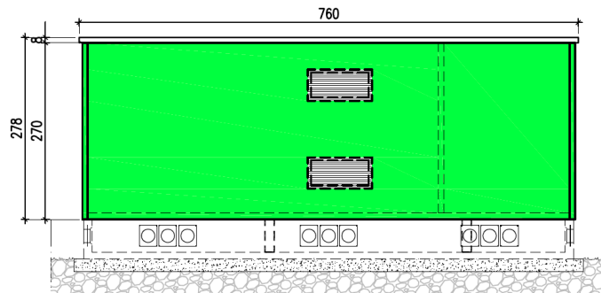
PROSPETTO P3
