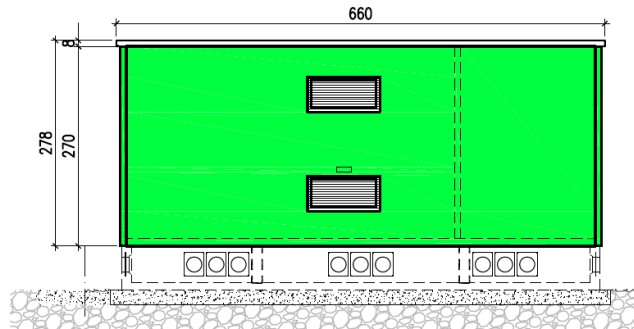
PROSPETTO P3
