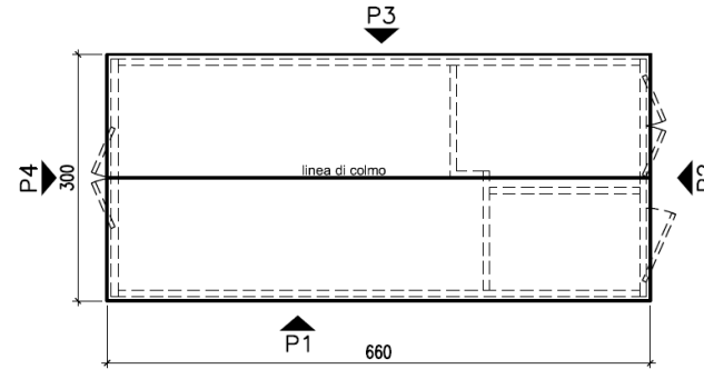
PIANTA COPERTURA
