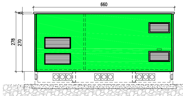
PROSPETTO P3
