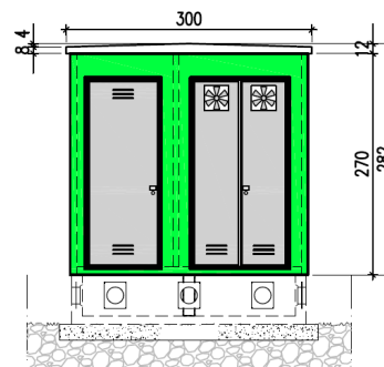
PROSPETTO P4
