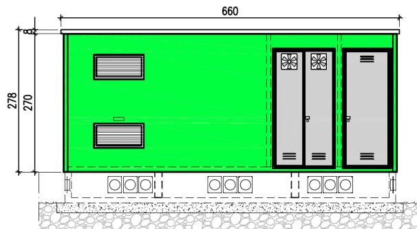
PROSPETTO P3
