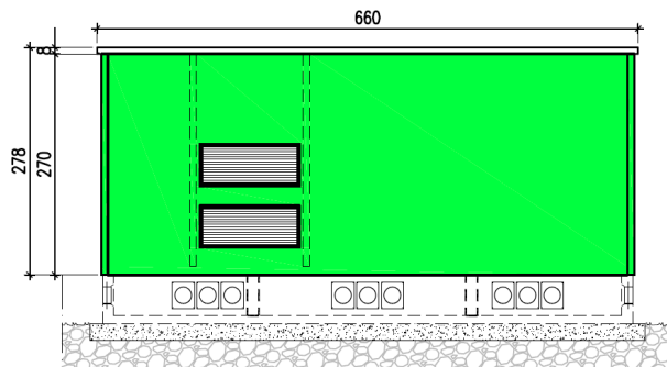
PROSPETTO P3
