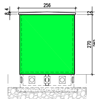
PROSPETTO P4
