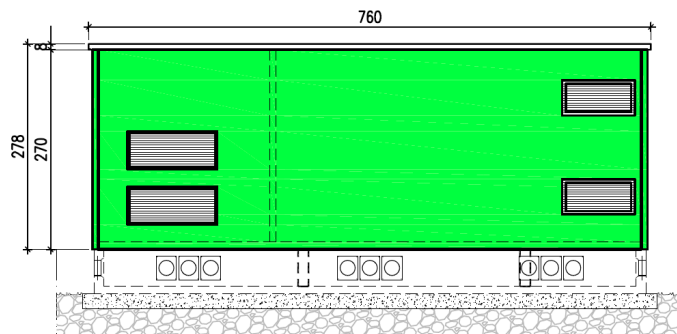
PROSPETTO P3
