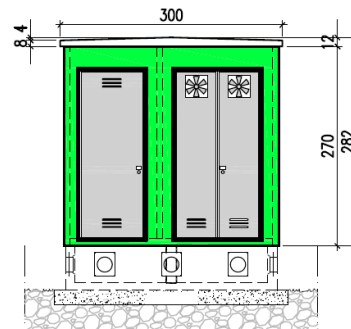
PROSPETTO P4
