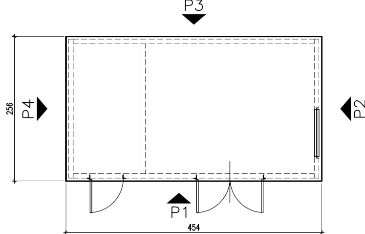
PIANTA COPERTURA
