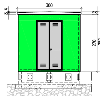
PROSPETTO P4
